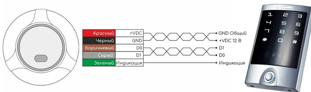
Рисунок 7. Рекомендуемая схема подключение по интерфейсу Wiegand
